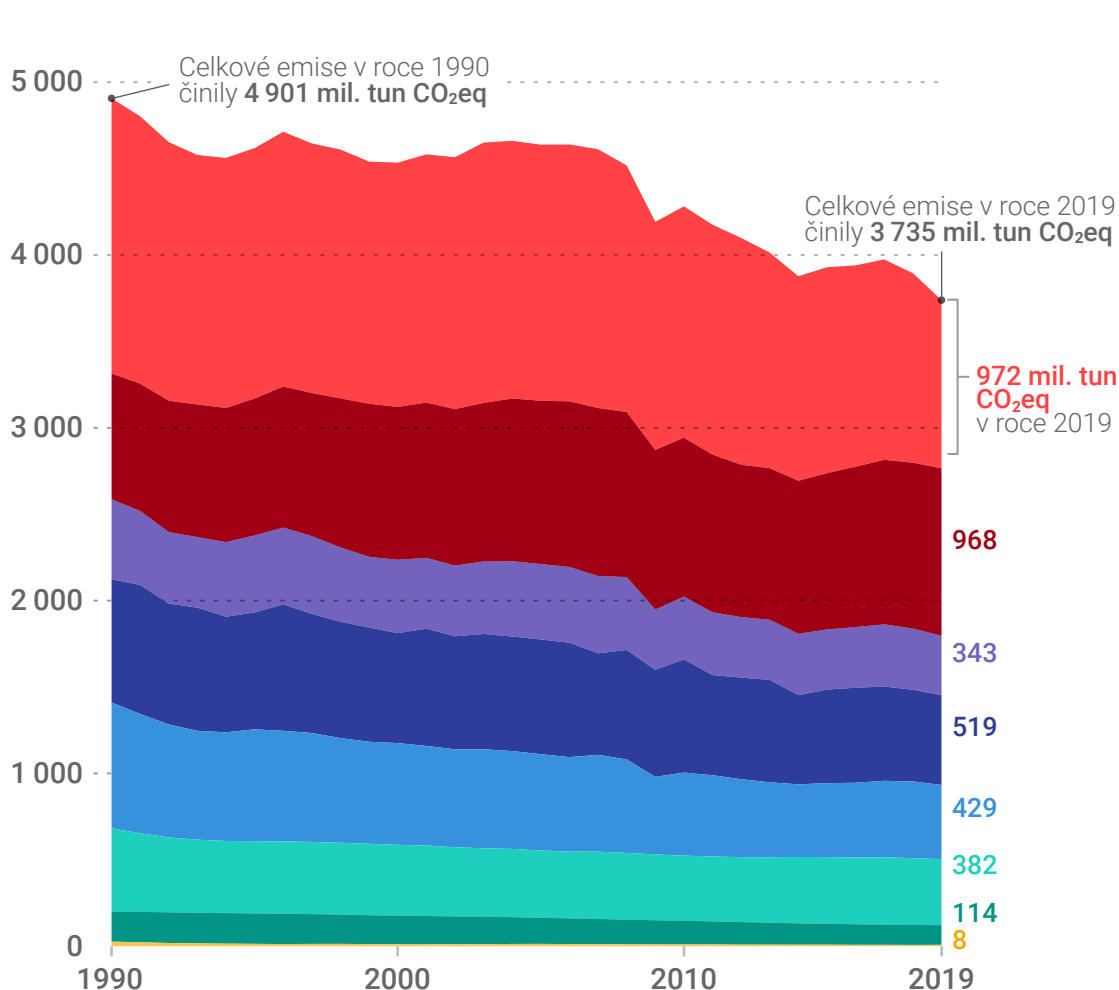
VÝVOJ EMISÍ V LETECH 1990–2019
